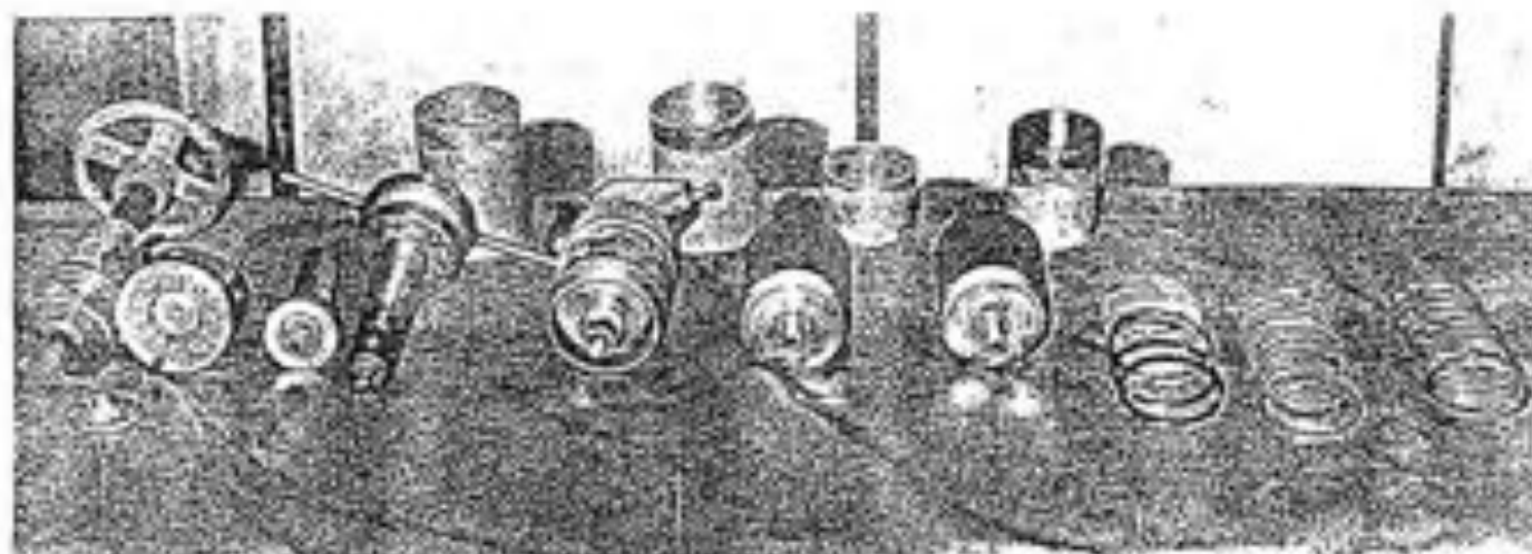
Dispositivo para el rectificado de las caras de los aros. Son aplicados en la reparación de motores de los autos LADA, MOSKVICH y FIAT. Introducir el cono mause 2 del dispositivo en el árbol principal de un torno. Este tiene una cavidad interior donde se coloca un abanico cónico, a través del cual se desplaza un tornillo, que acciona sobre dicha cavidad, el que permite la fijación del aro después de cortado para dar terminación por las caras a los aros y, a su vez, hacer el raspador a los aros de compresión, Pinar del Río, Pinar del Río.
