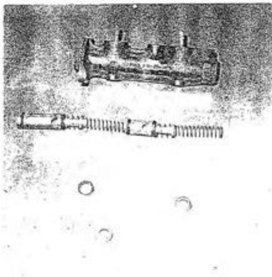
Modificación de la bomba de freno del auto LADA. Guimaro, Camagüey.
